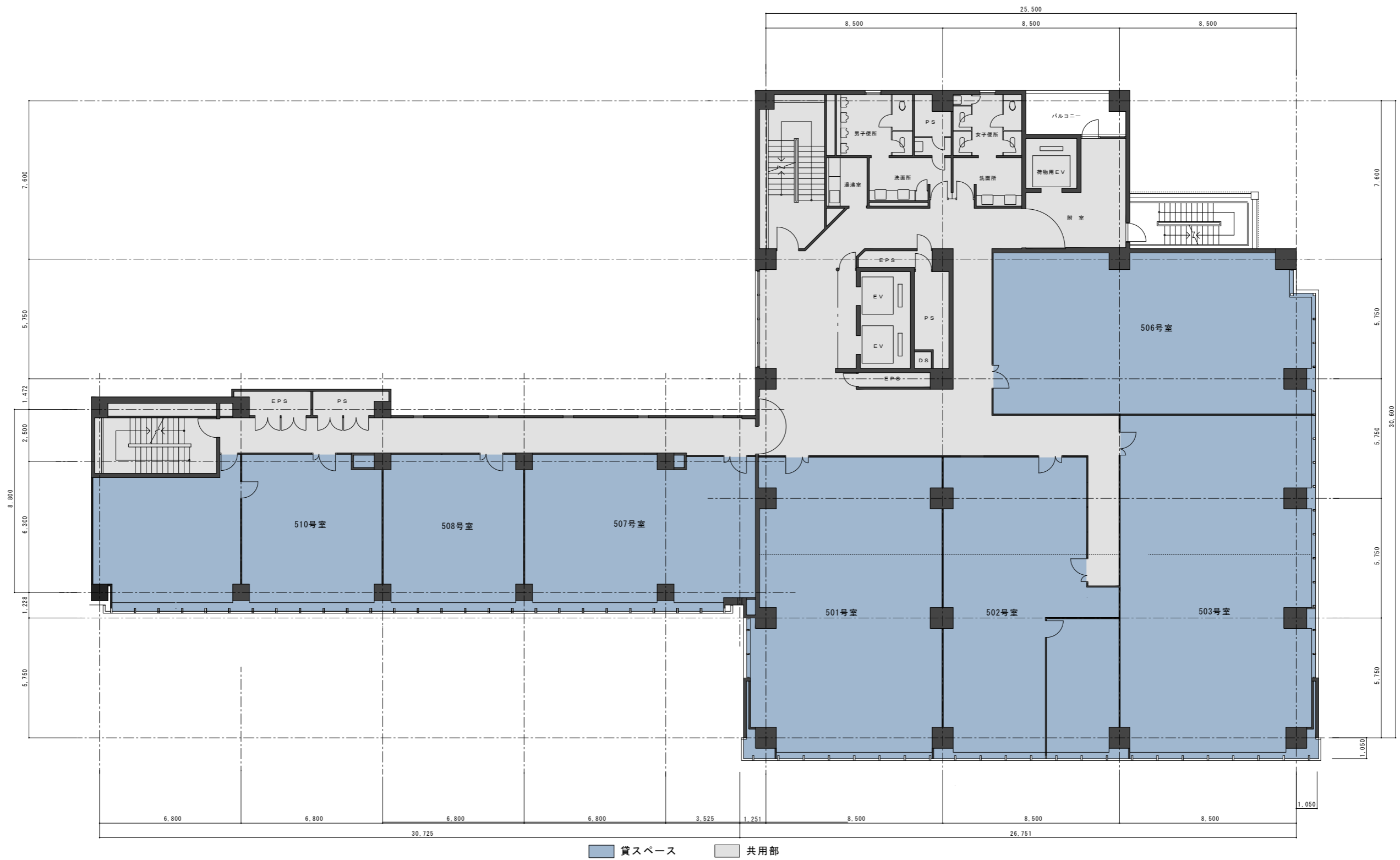
5階平面図
