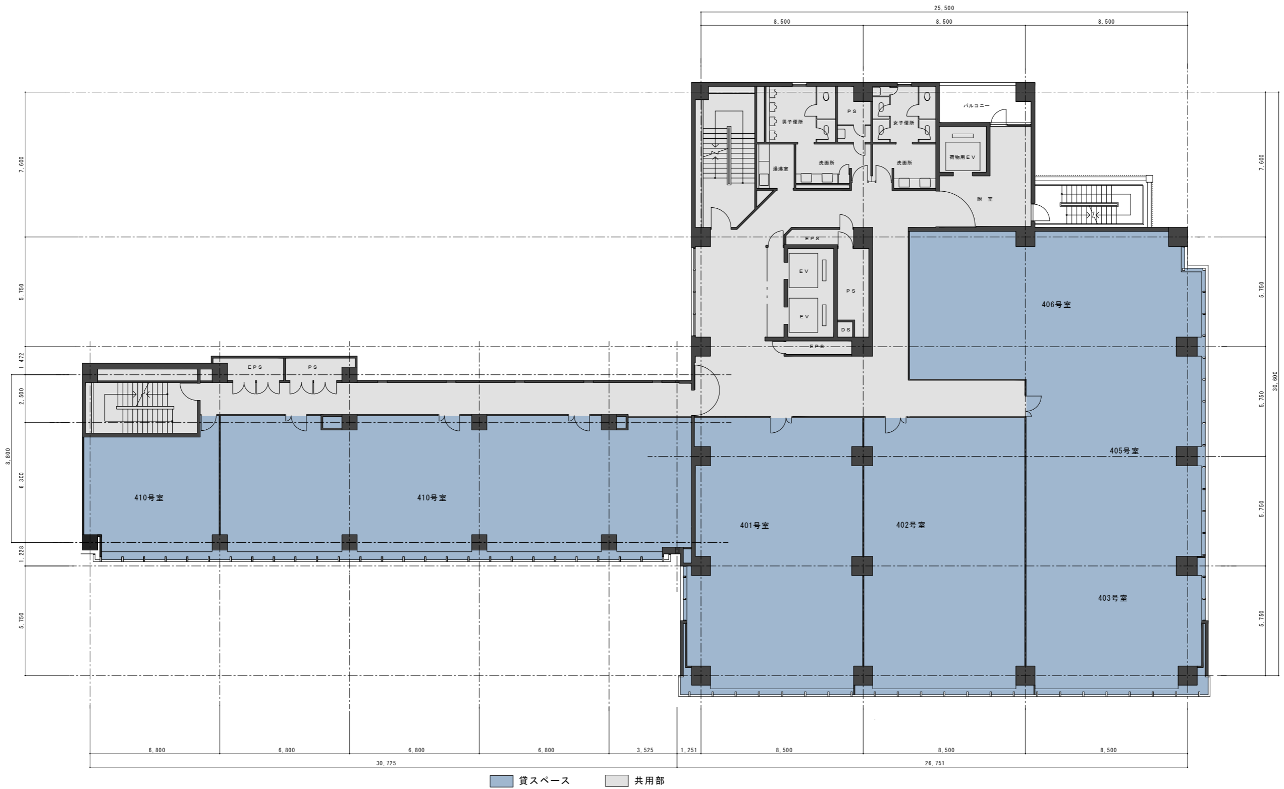
4 階 平 面 図
